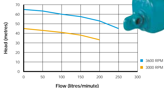
Blazemaster B55H
